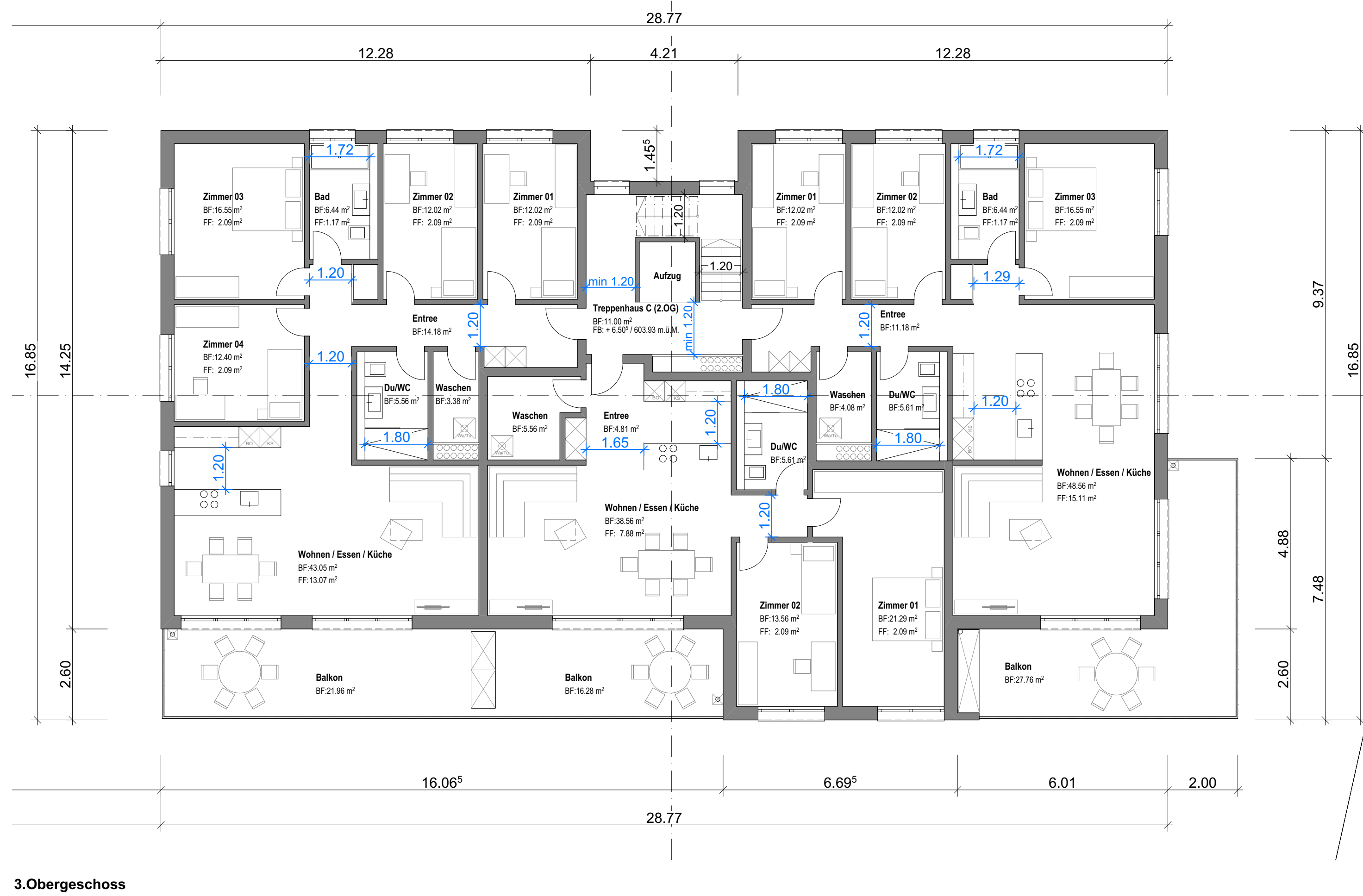
3.Obergeschoss
