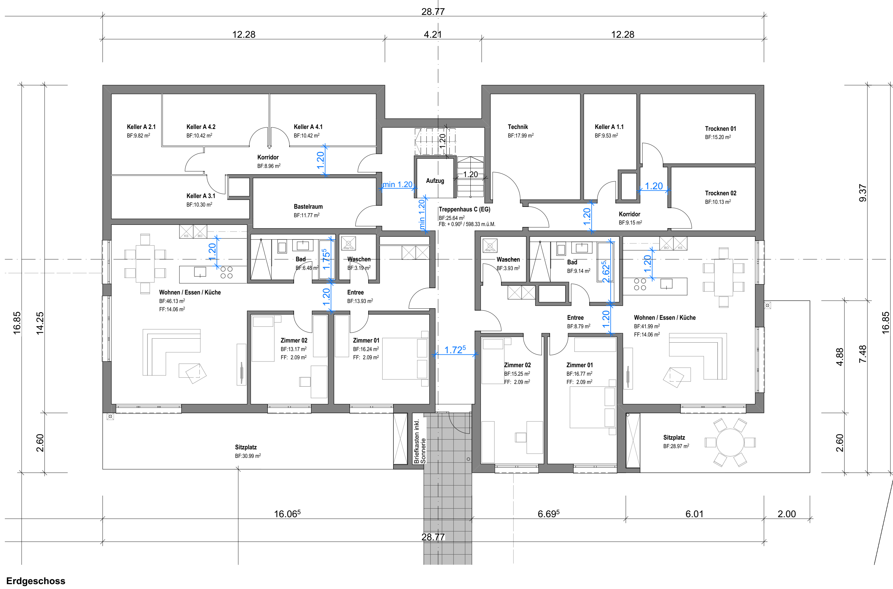
Erdgeschoss
