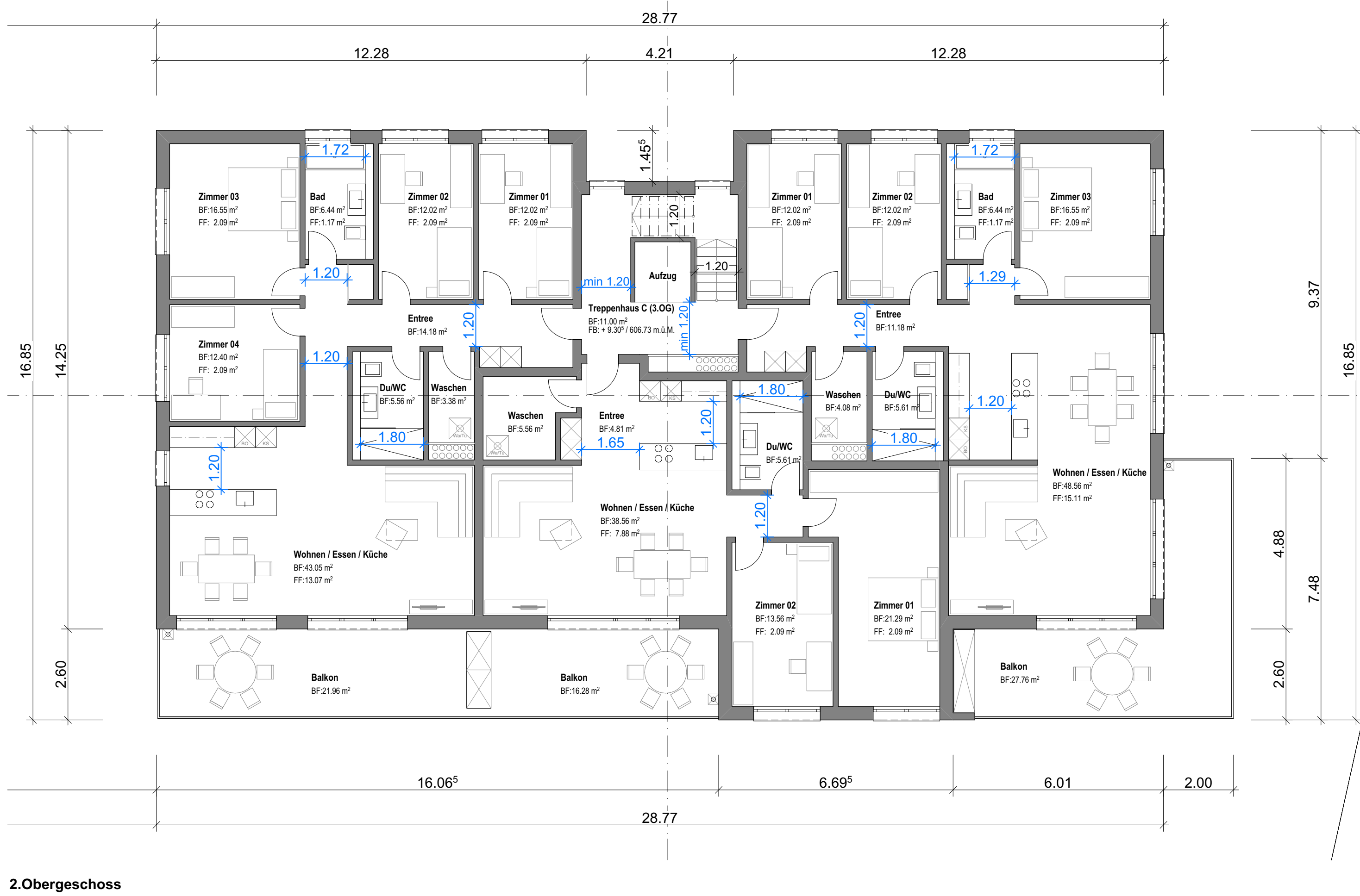
2.Obergeschoss
