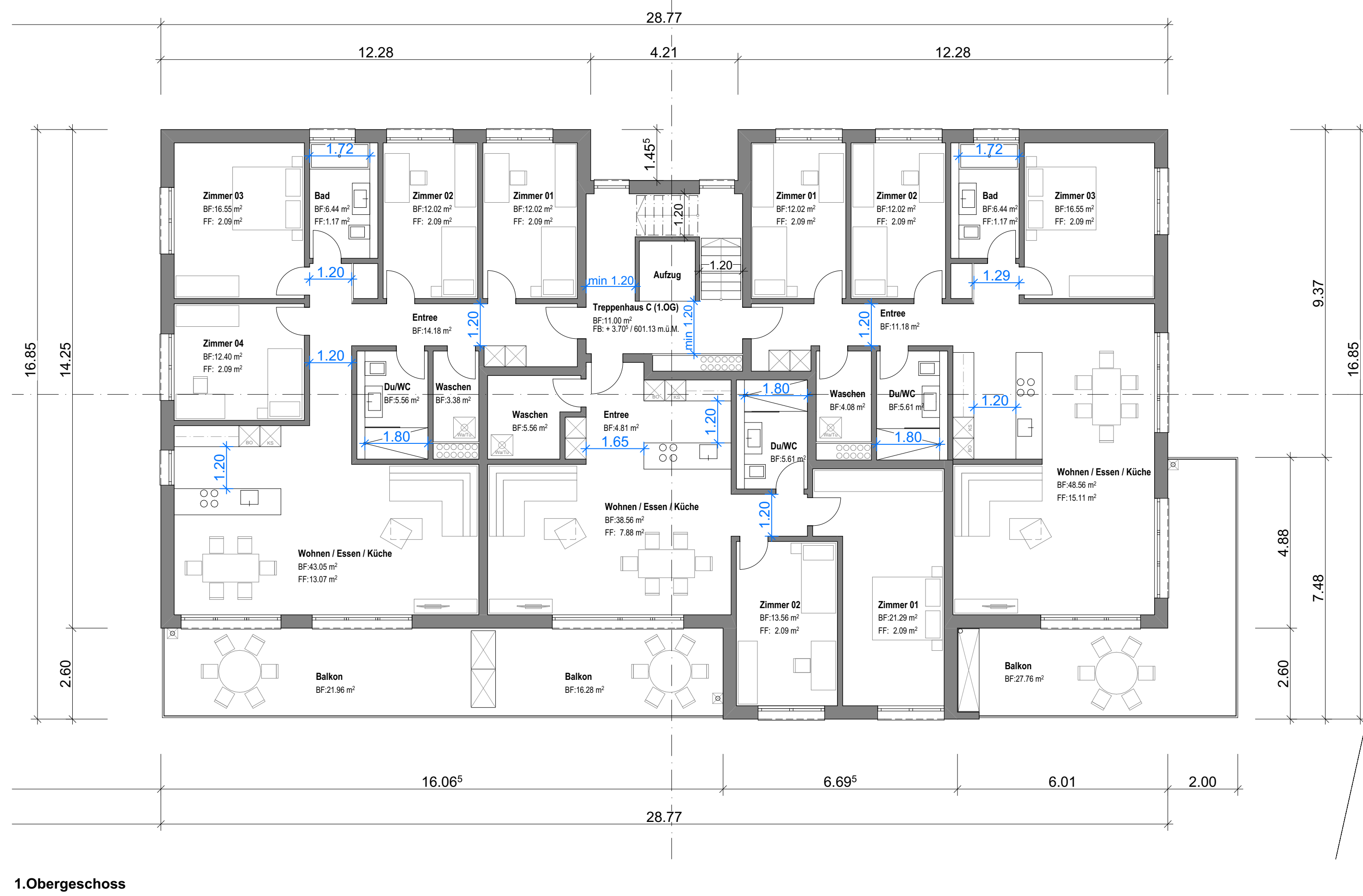
1.Obergeschoss
